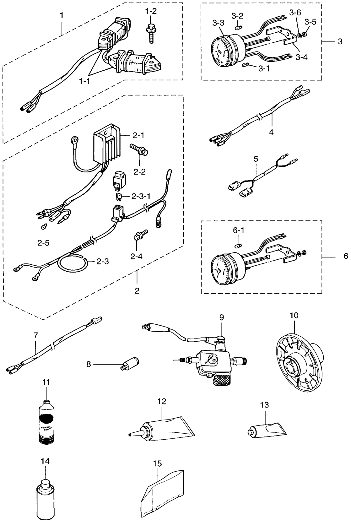
Fig. 21 オプションパーツ (アクセサリ) OPTIONAL PARTS (ACCESSORIES)
