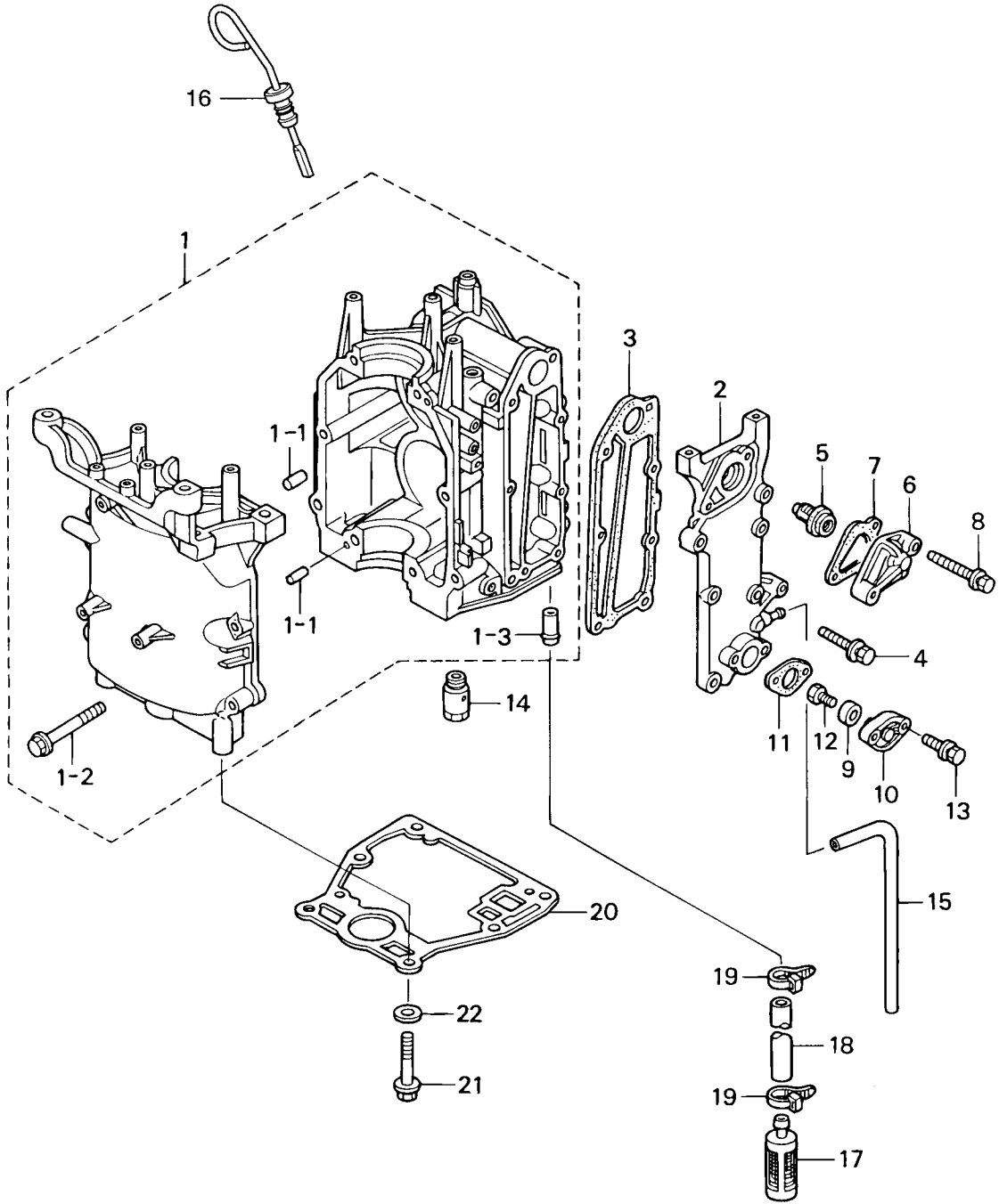
シリンダ CYLINDER Fig. 2
