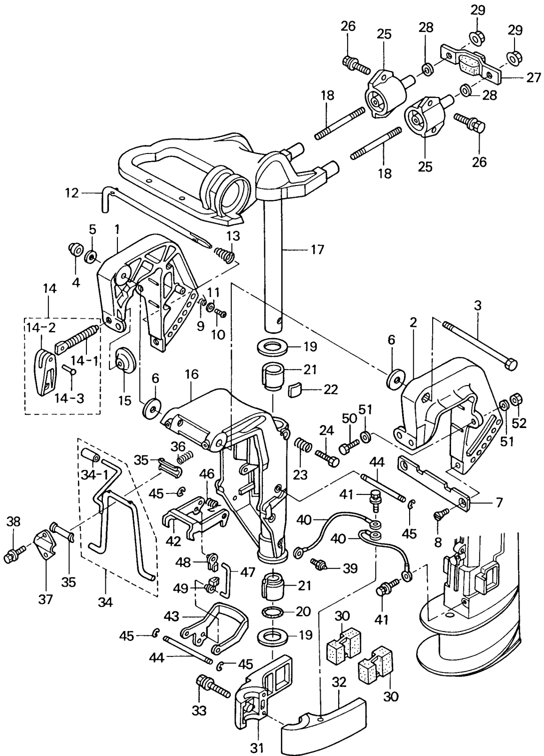
Fig. 17A ブラケット (Fタイプ) BRACKET (for "F" Type)
