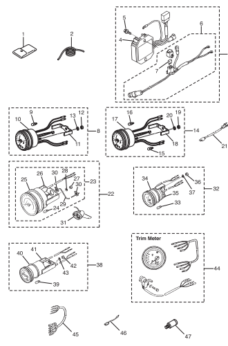
Fig. 23 OPTIONAL PARTS · ACCESSORI オプションパーツ・アクセサリ
