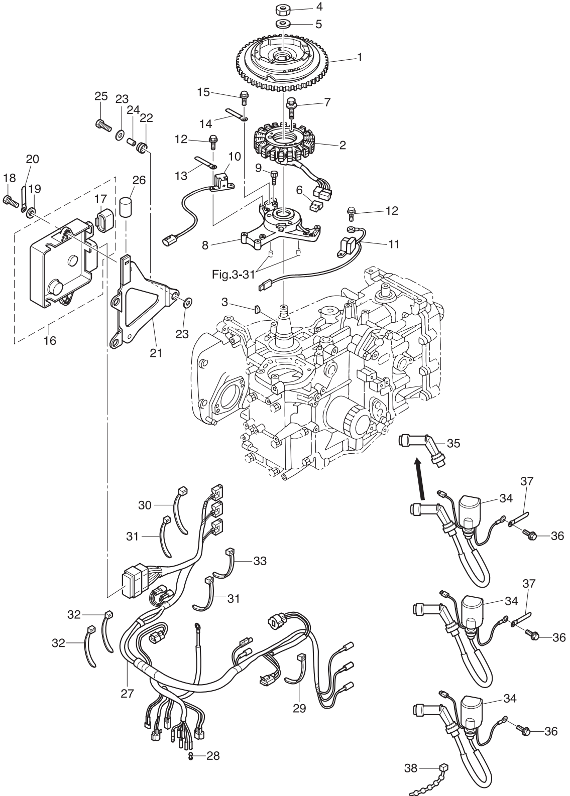
Fig. 8 MAGNETO マグネト
