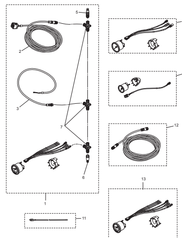
Fig. 26 OPTIONAL PARTS (4) オプションパーツ (4)
