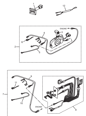
Fig. 27 RIGGING KIT リギングキット
