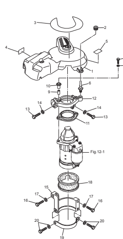
Fig. 11 ELECTRIC PARTS (STARTER MOTOR) (1) エレクトリックパーツ (スタータモータ) (1)
