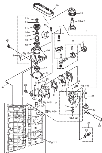
Fig. 8 VAPOR SEPARATOR · FUEL LINE ベーパーセパレータ・フエルのライン
