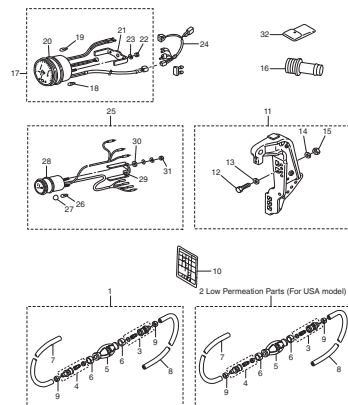
リギングキット Fig. 24 RIGGING KIT
