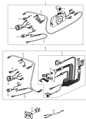
リモコンボックス構成部品 Fig. 27 COMPONENT PARTS OF REMOTE CONTROL BOX
