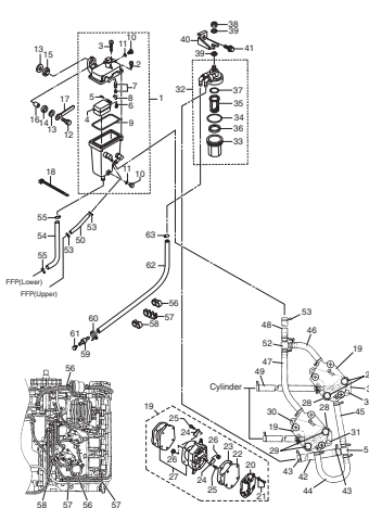
ベーパーセパレータ & フエエルライン Fig. 8 VAPOR SEPARATOR & FUEL LINE
