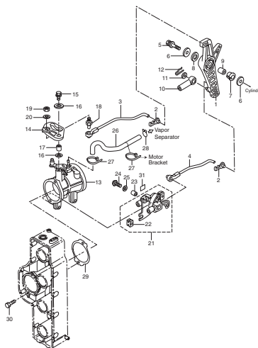
スロットル Fig. 7 THROTTLE
