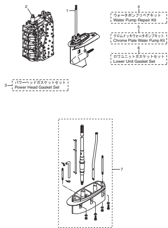
アセンブリキット Fig. 26 ASSEMBLY KIT
