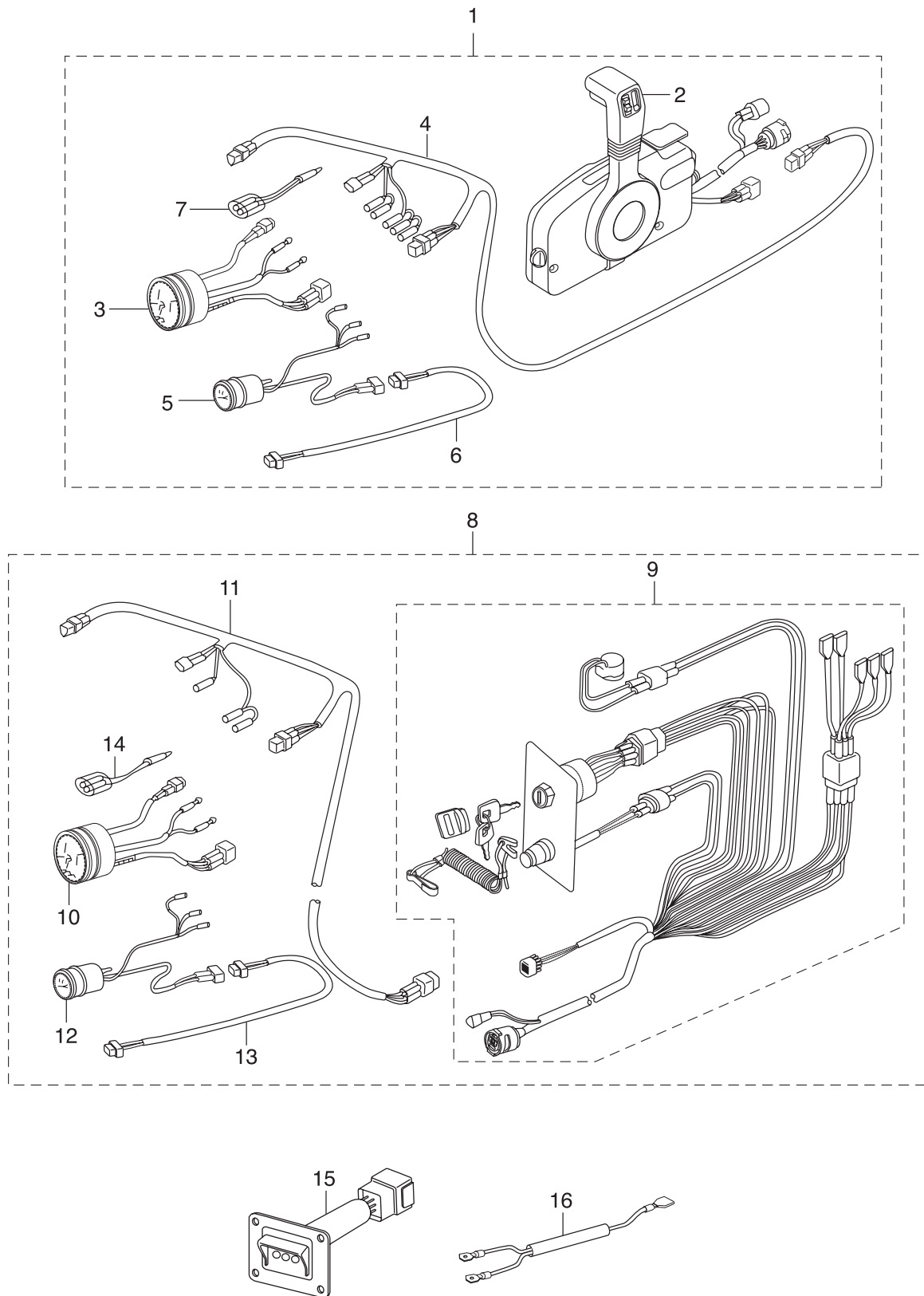
リギングキット Fig. 24 RIGGING KIT
