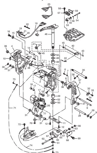
ブラケット Fig. 16 BRACKET
