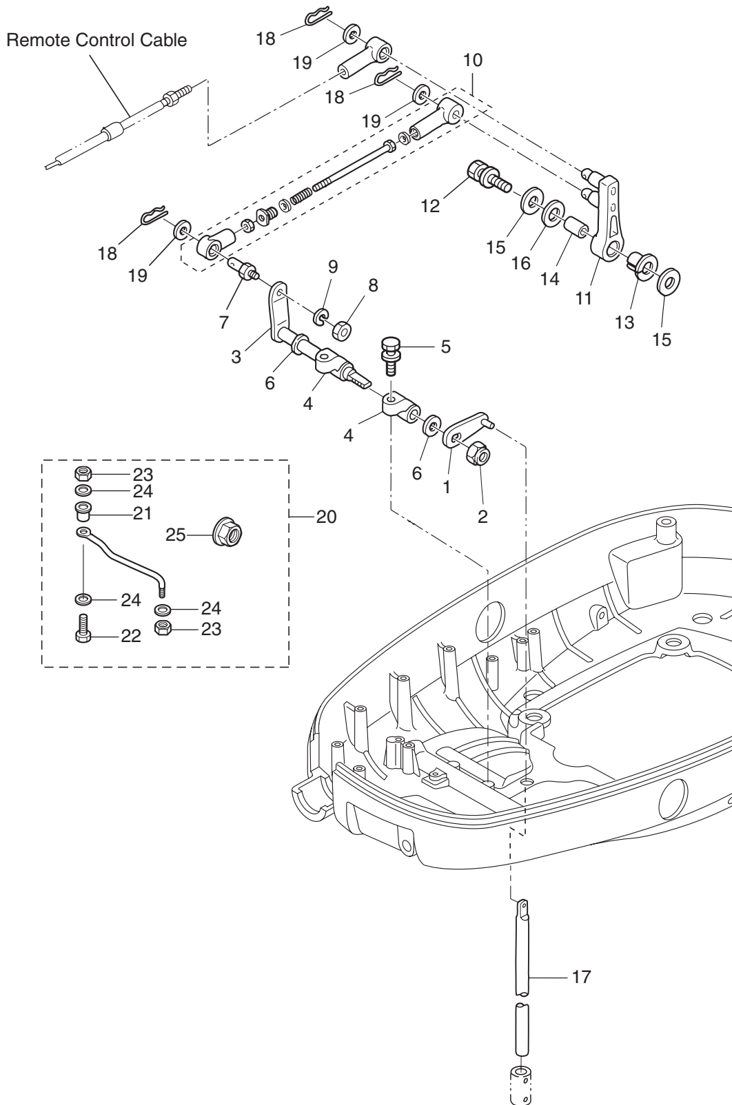
シフト Fig. 19 SHIFT
