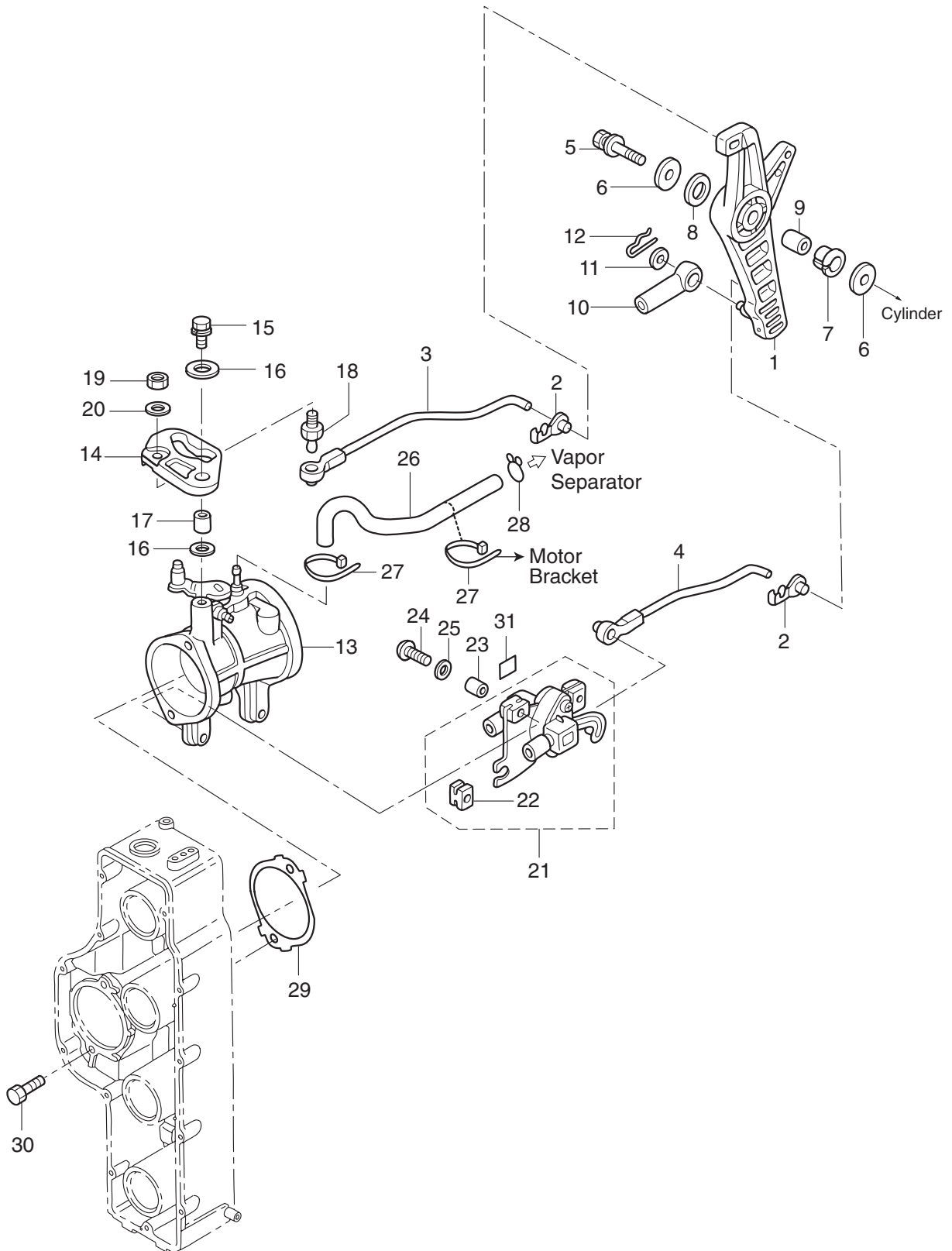
スロットル Fig. 7 THROTTLE
