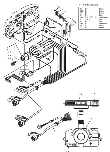
リモコンボックス構成部品 (電装品関係) Fig. 28 COMPONENT PARTS OF REMOTE CONTROL BOX (ELECTRICAL PARTS)
