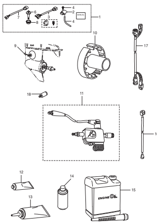
オプションパーツ (3) Fig. 25 OPTIONAL PARTS (3)
