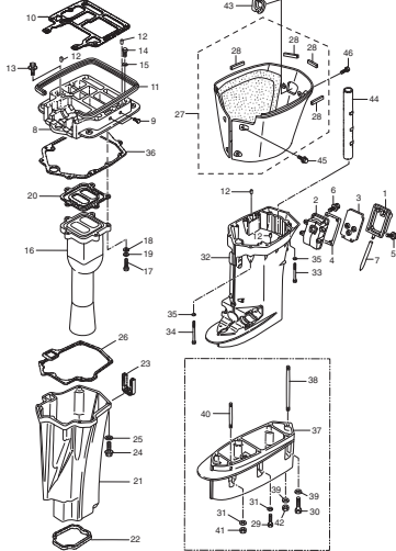
ブラケット Fig. 16 BRACKET
