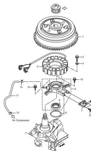
マグネト Fig. 9 MAGNETO
