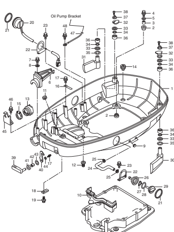
ボトムカウル Fig. 18 BOTTOM COWL
