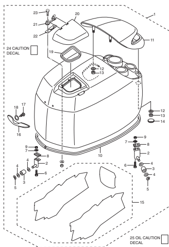
オプションパーツ (2) Fig. 23 OPTIONAL PARTS (2)
