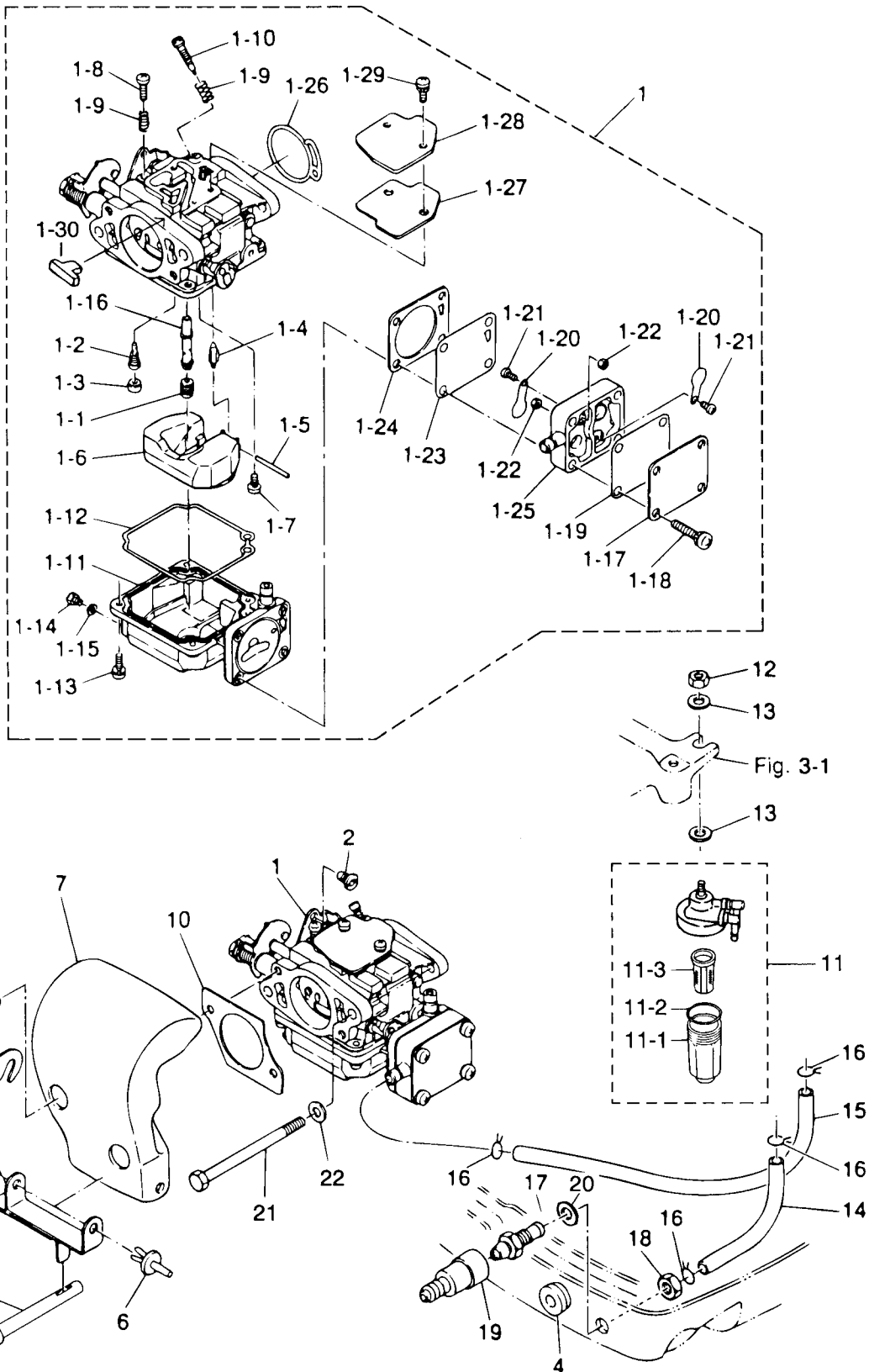
キャブレタ・フエエルフィルタ Fig. 4 CARBURETOR · FUEL FILTER
