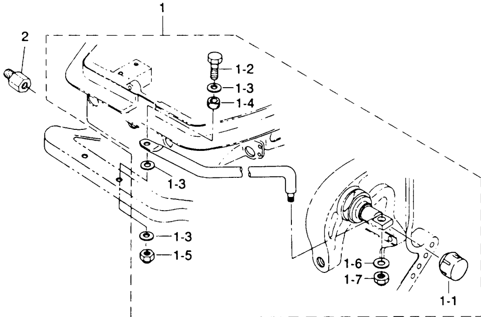
Fig. 16 オプションパーツドラックリンク/リバースロック OPTIONAL PARTS DRAG LINK/REVERS LOCK
