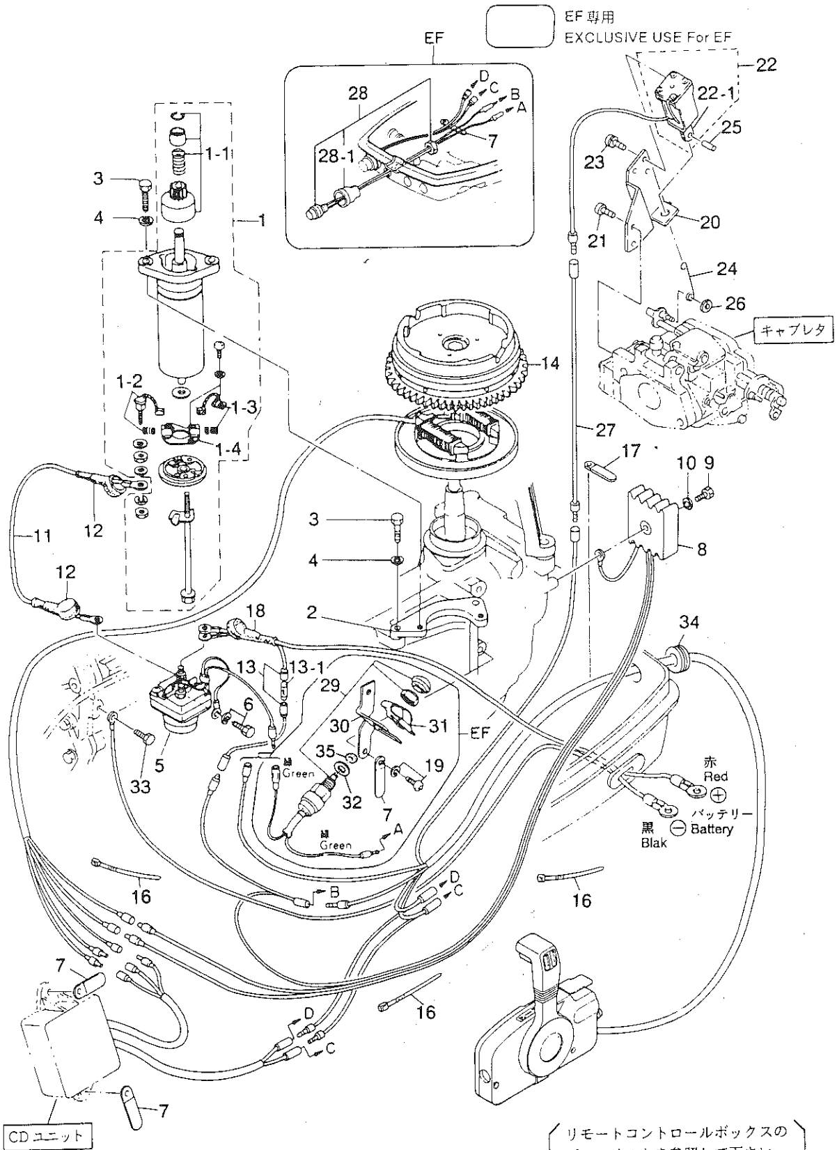
オプションパーツエレクトリックスタータ Fig. 17 POTENTIAL PARTS ELECTRIC STARTER
