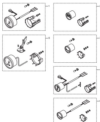
Fig. 31 ASSEMBLY · KIT PARTS アセンブリ・キットパーツ
