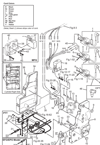
Fig. 9 ELECTRIC PARTS (C.D. UNIT) エレクトリックパーツ (C.D. ユニット)
