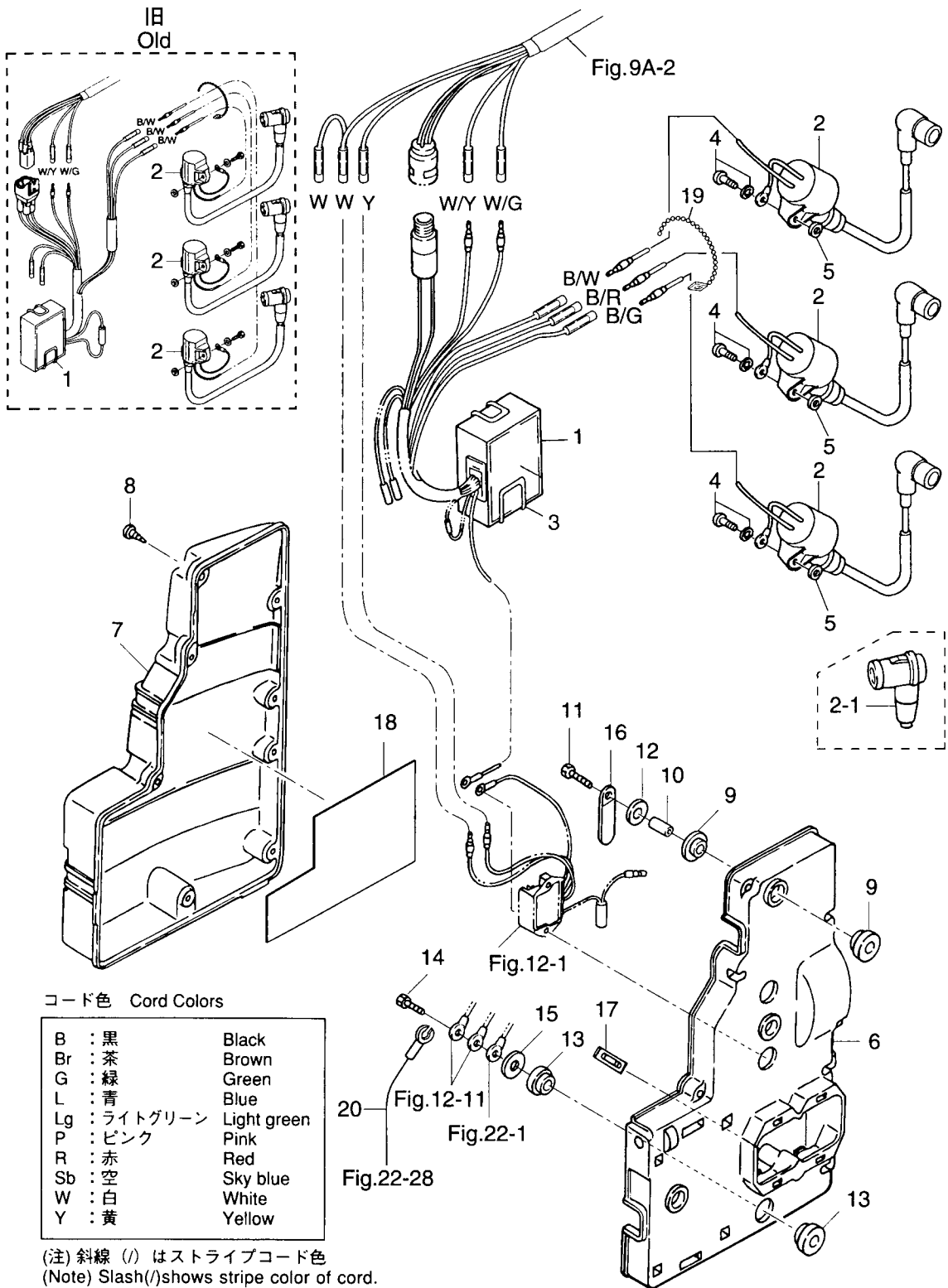
エレクトリックパーツ (C.D. ユニット) Fig. 10 ELECTRIC PARTS (C.D. UNIT)
