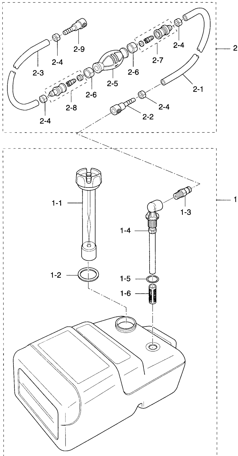
セパレートフュエルタンク Fig. 24 SEPARATE FUEL TANK
