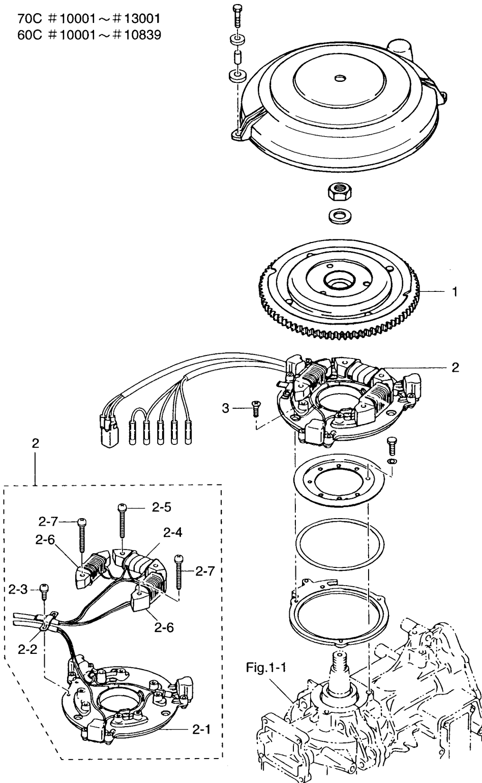
Fig. 9B マグネト (旧) MAGNETO (Old)
