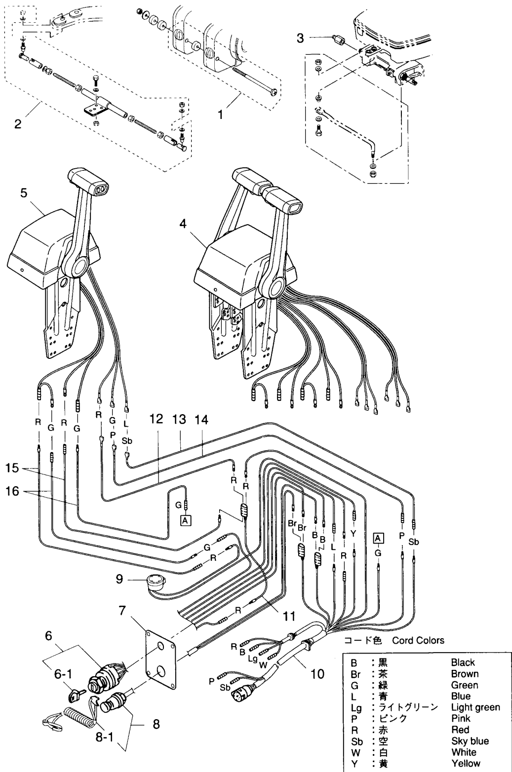
Fig. 27 オプショナルパーツ (2) OPTIONAL PARTS (2)
