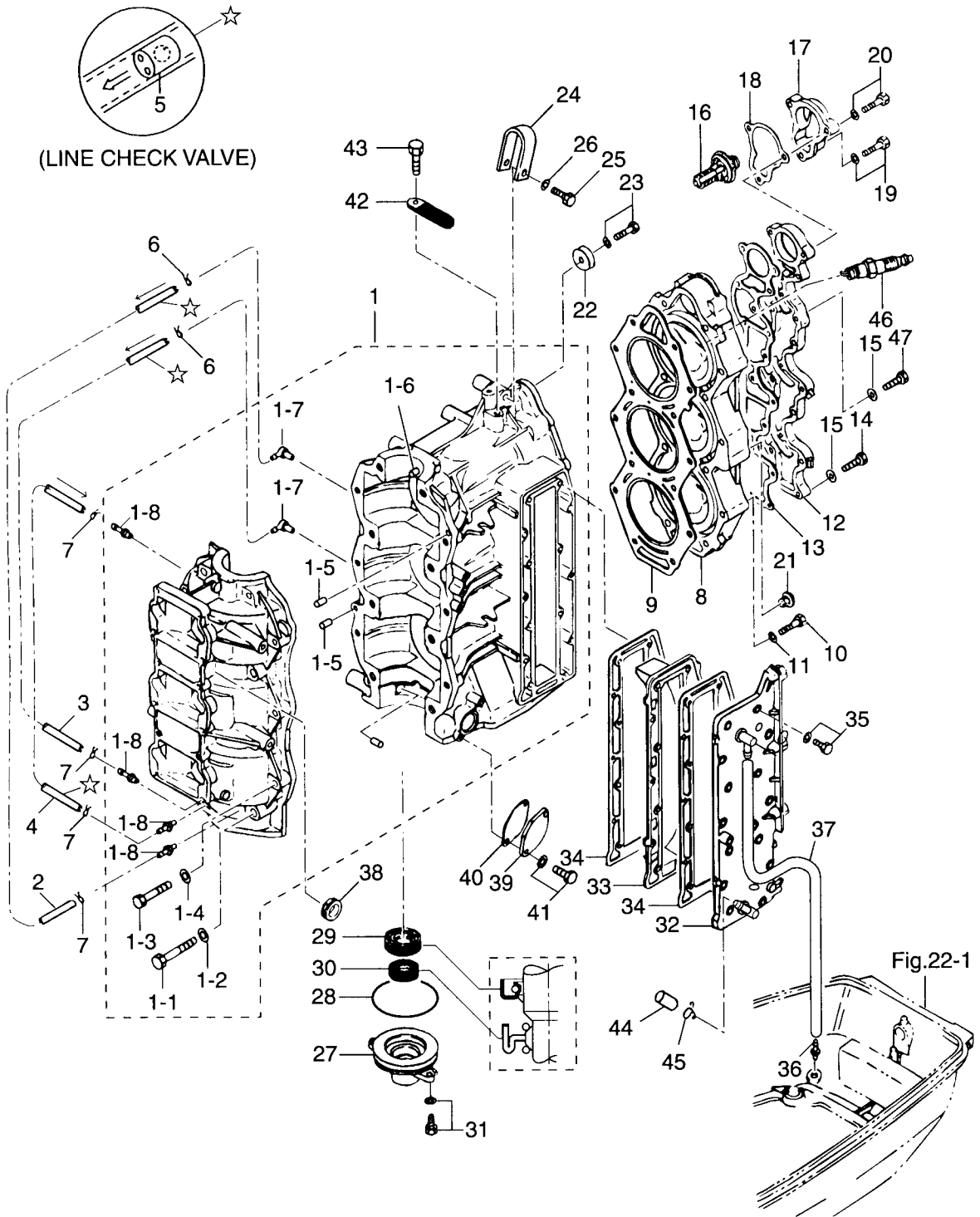
シリンダ・クランクケース CYLINDER · CRANK CASE Fig. 1
