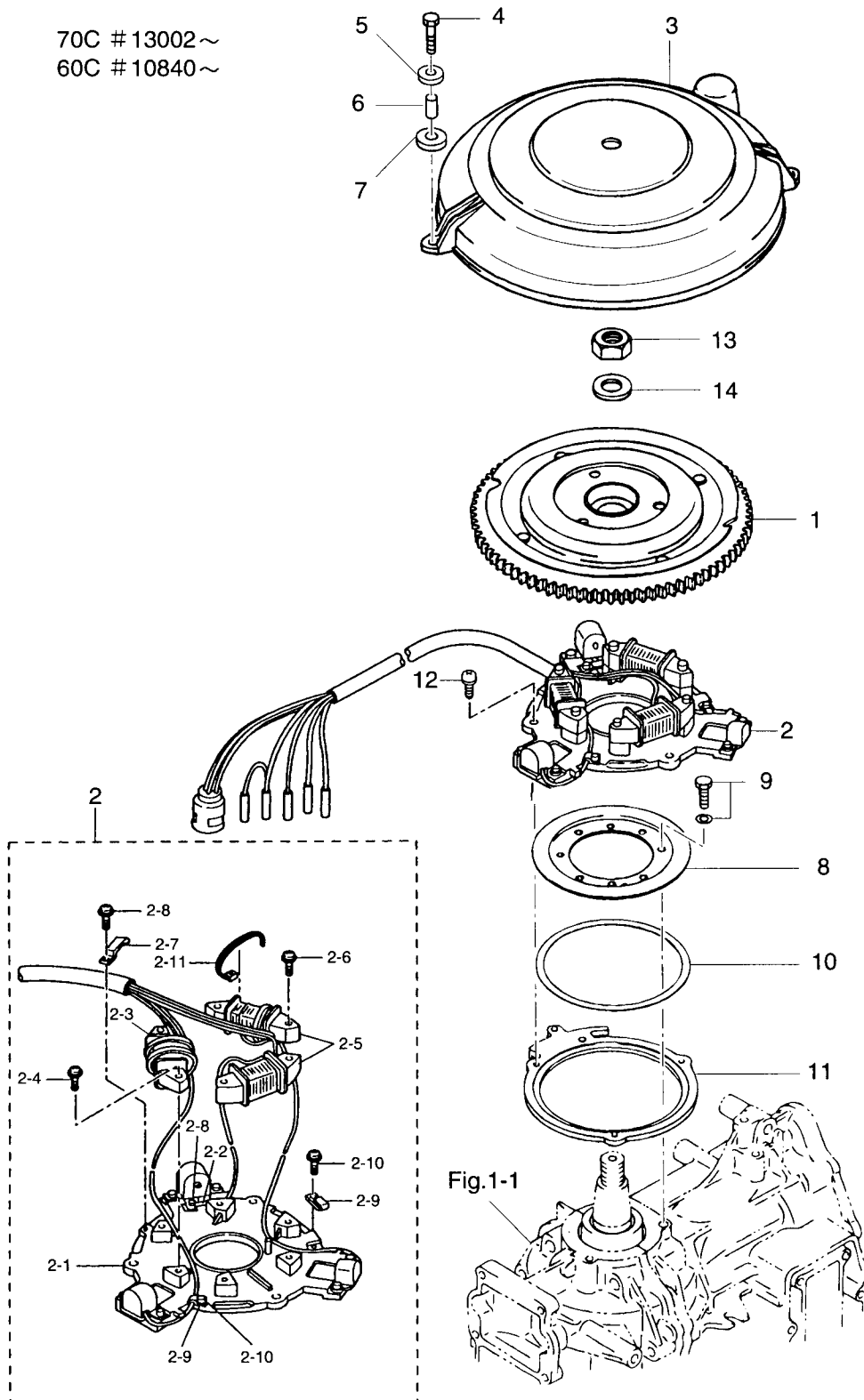
Fig. 9A マグネット (新) MAGNETO (New)
