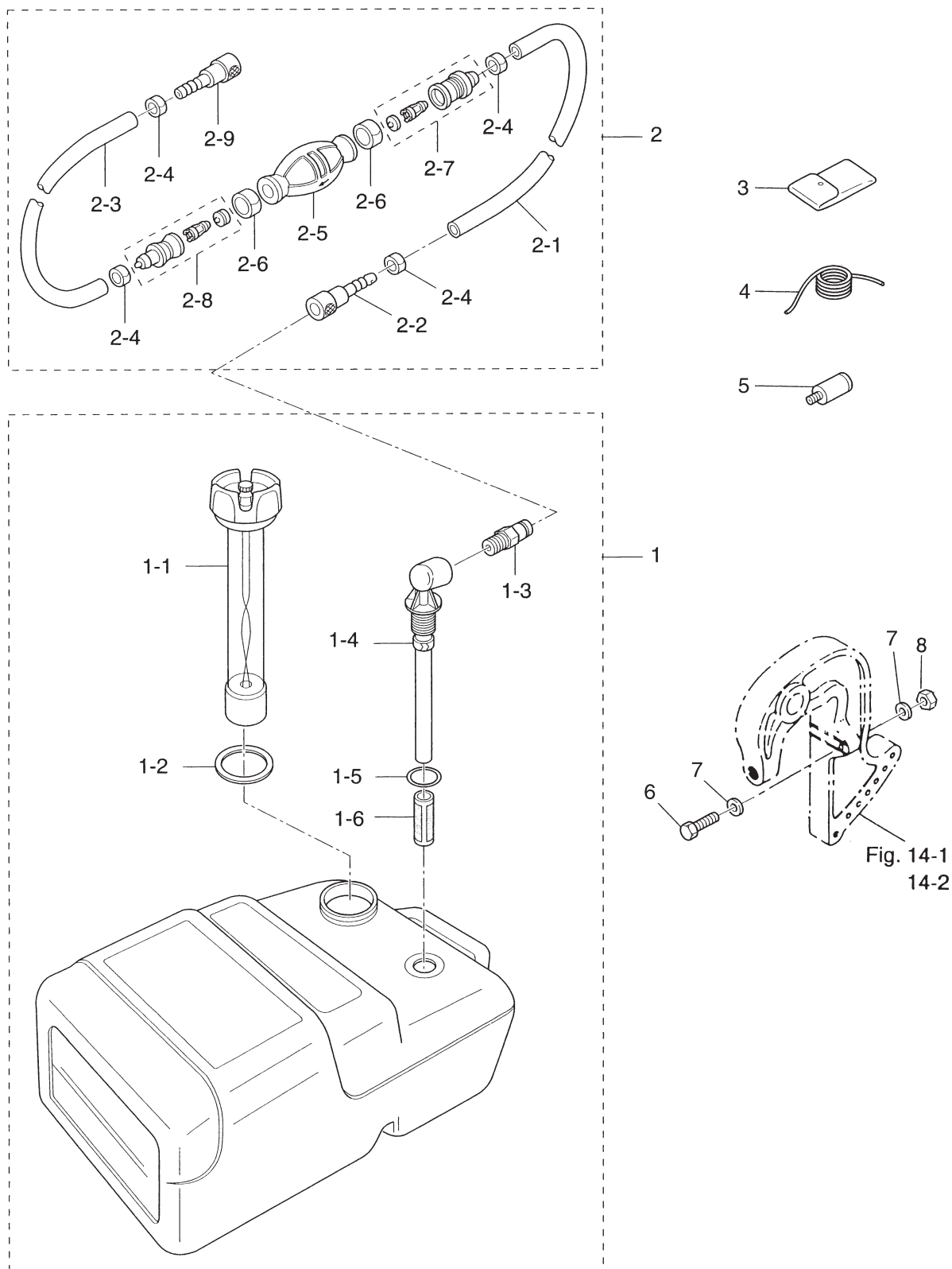
Fig. 17 セパレートフュエルタンク(プラスチック)・アクセサリー SEPARATE FUELE TANK (PLASTIC) · ACCESSORIES
