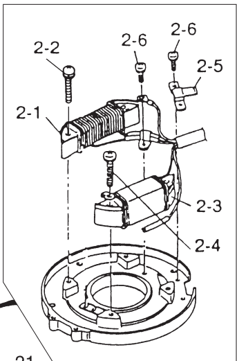
マグネト MAGNETO
