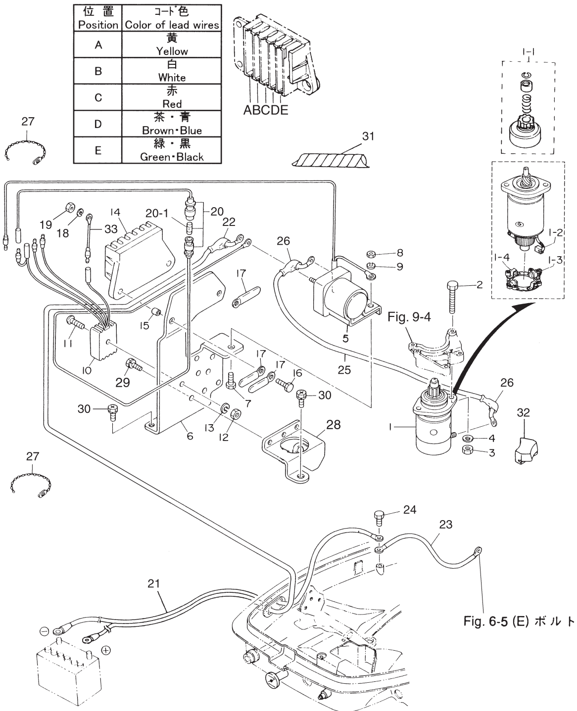
Fig. 19 オプションパーツ (II) エレクトリックスタータ (P, F タイプ共通) OPTIONAL PARTS (II) ELECTRIC STARTER (Common use for P & F types)
