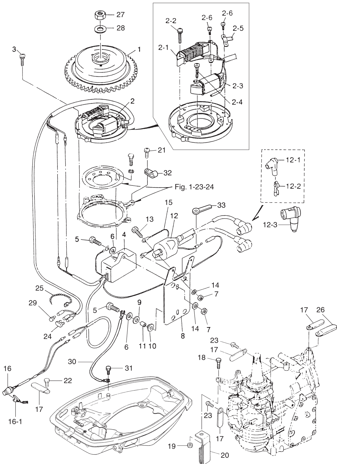
Fig. 6 マグネト 25C3 #50039 ~ MAGNETO 30A4 #35175 ~
