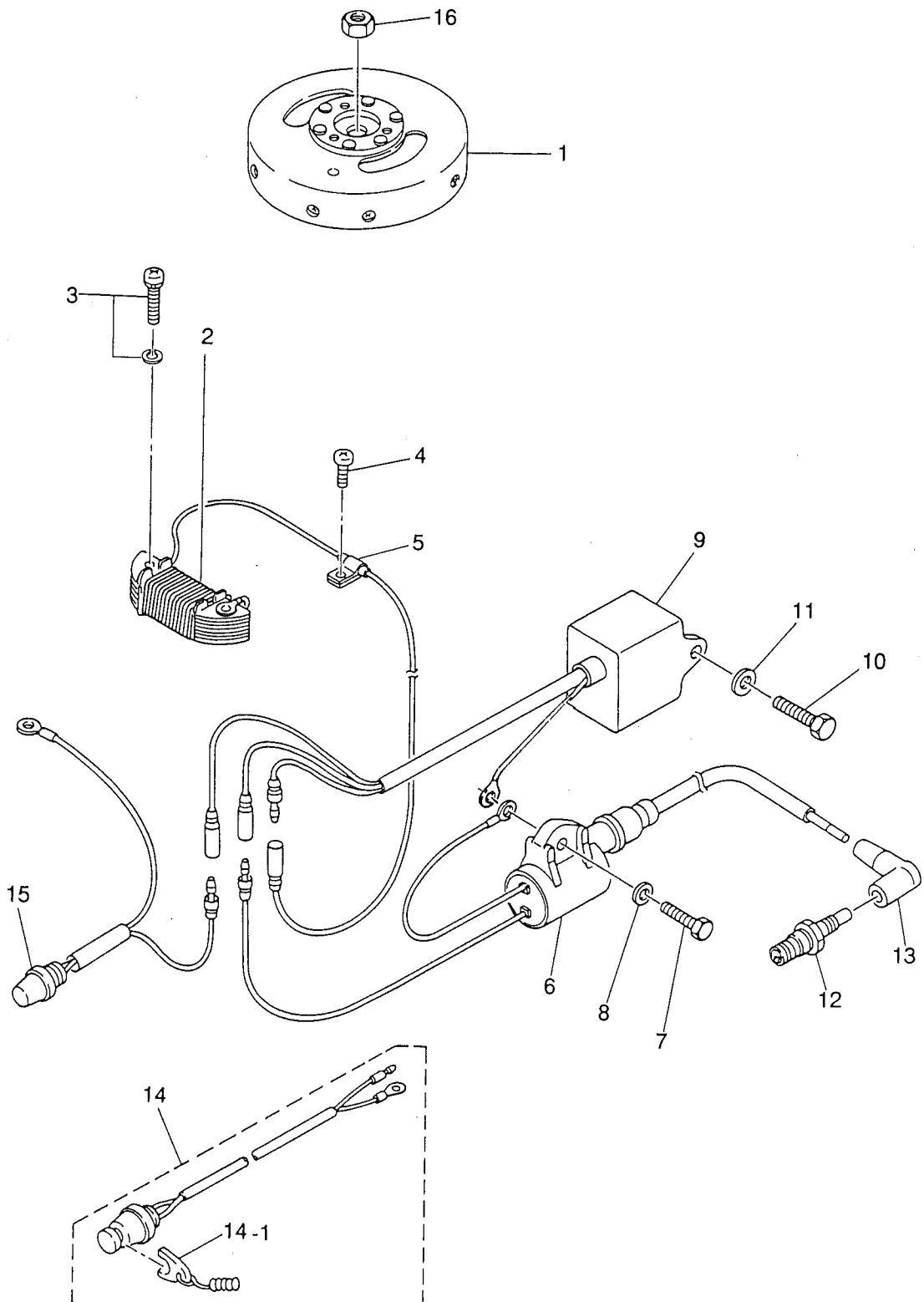
Fig. 3 マグネト MAGNETO
