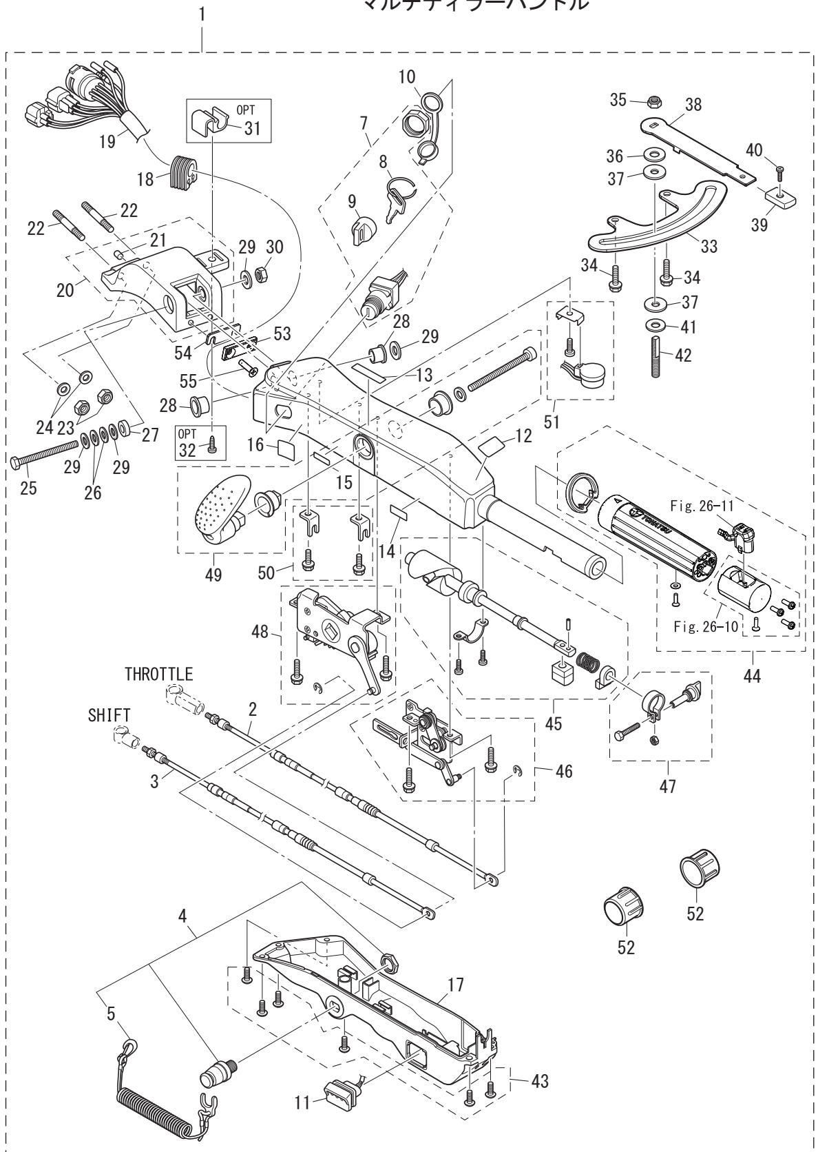
Fig. 20 MULTI TILLER HANDLE マルチティラーハンドル
