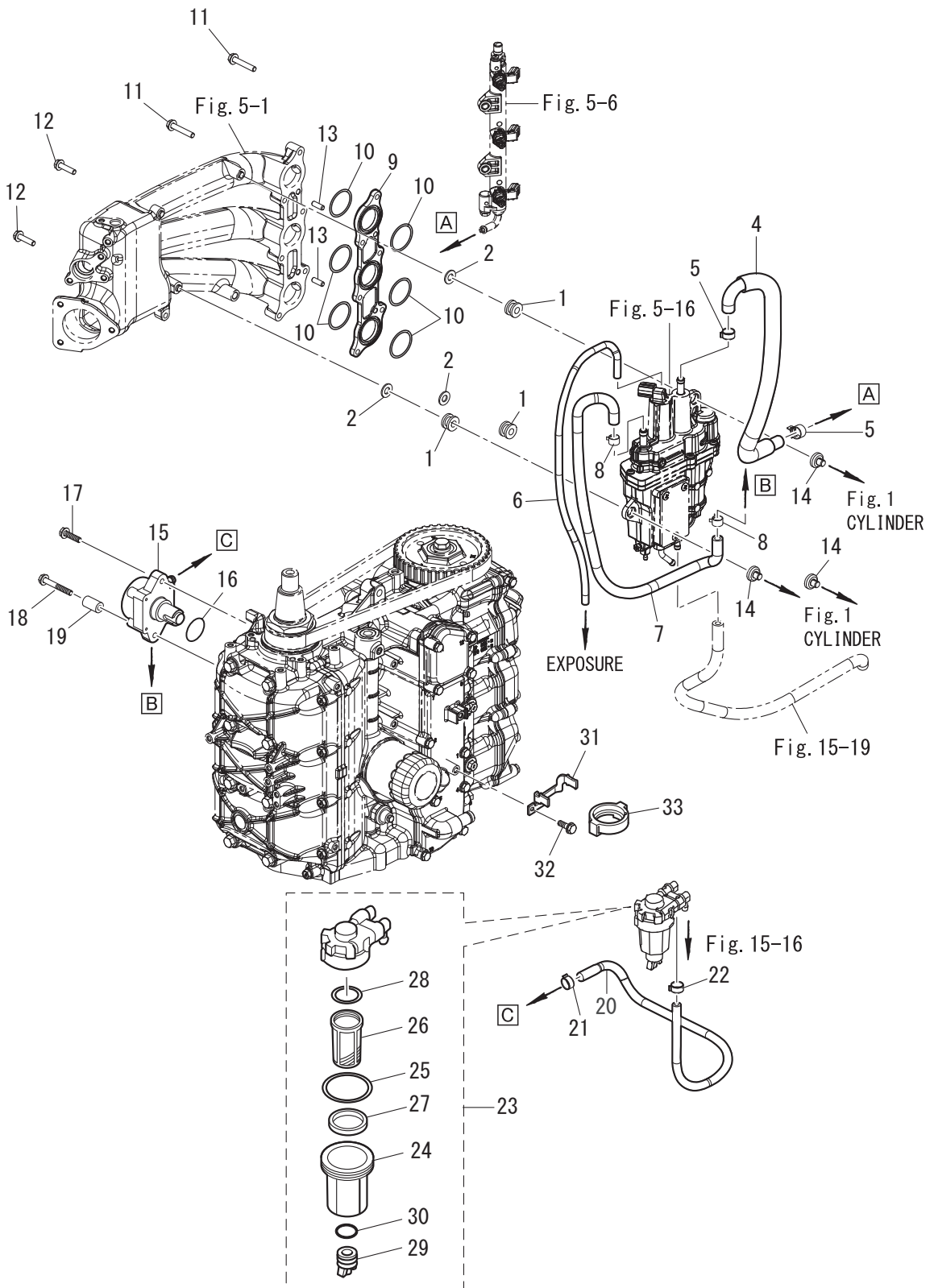
Fig. 6 FUEL SYSTEM フュエルシステム
