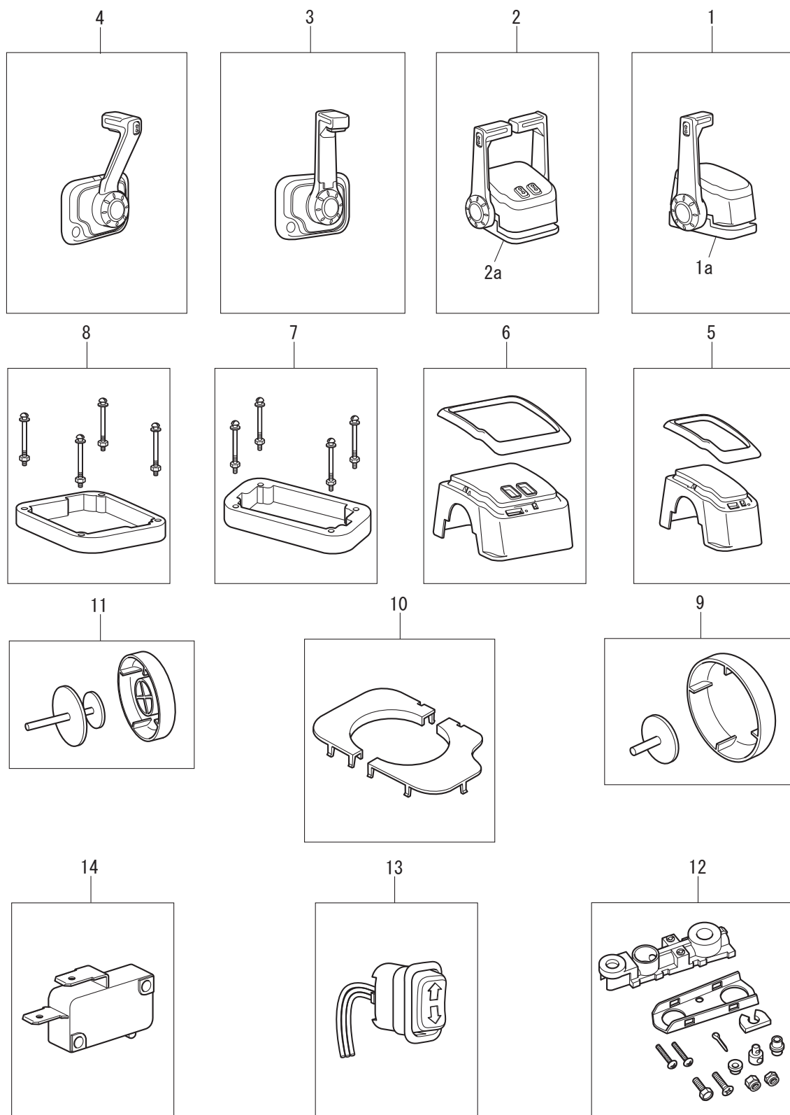
Fig. 24 OPTIONAL PARTS (2) オプションパーツ (2)
