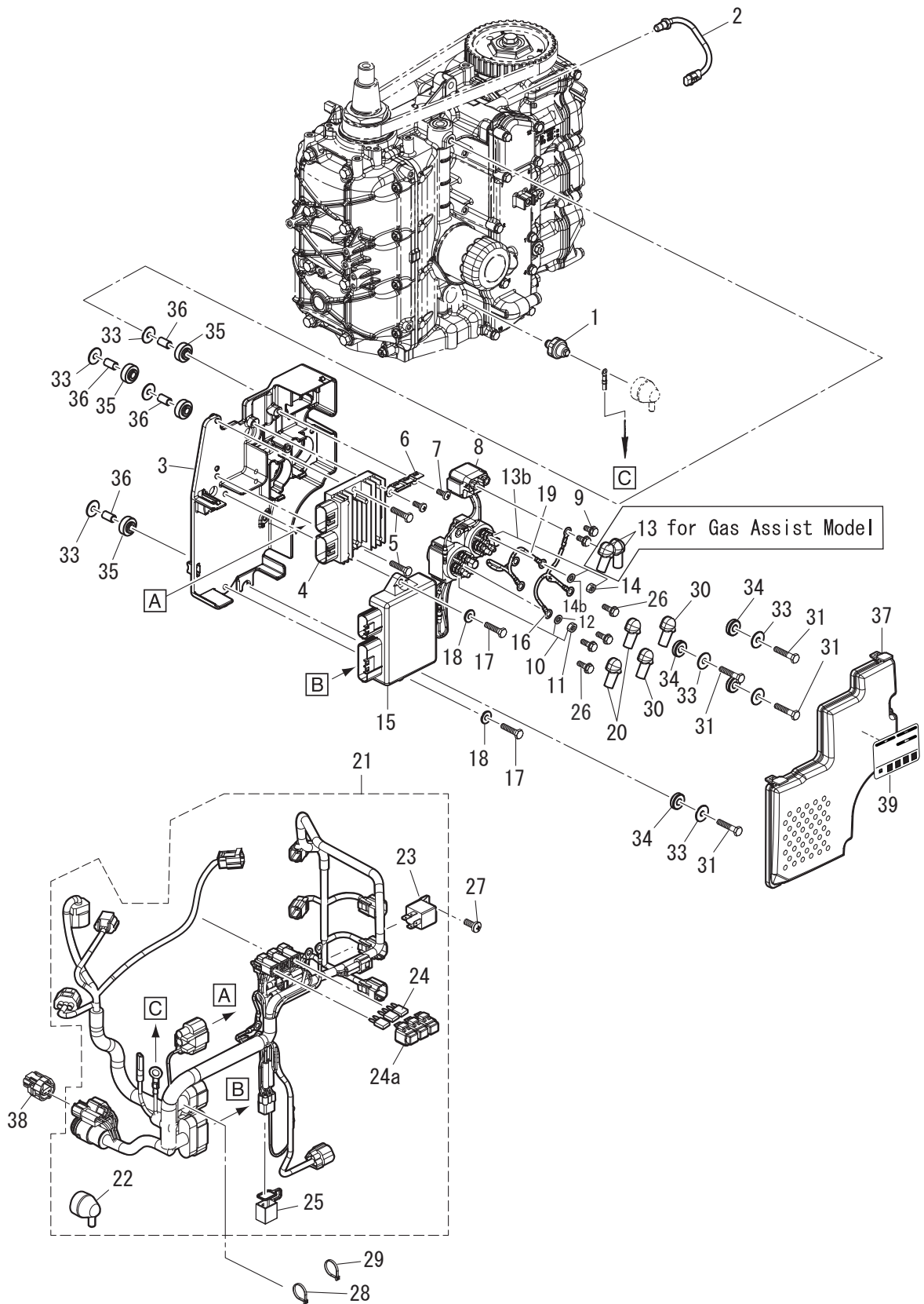
Fig. 9 ELECTRIC PARTS エレクトリックパーツ
