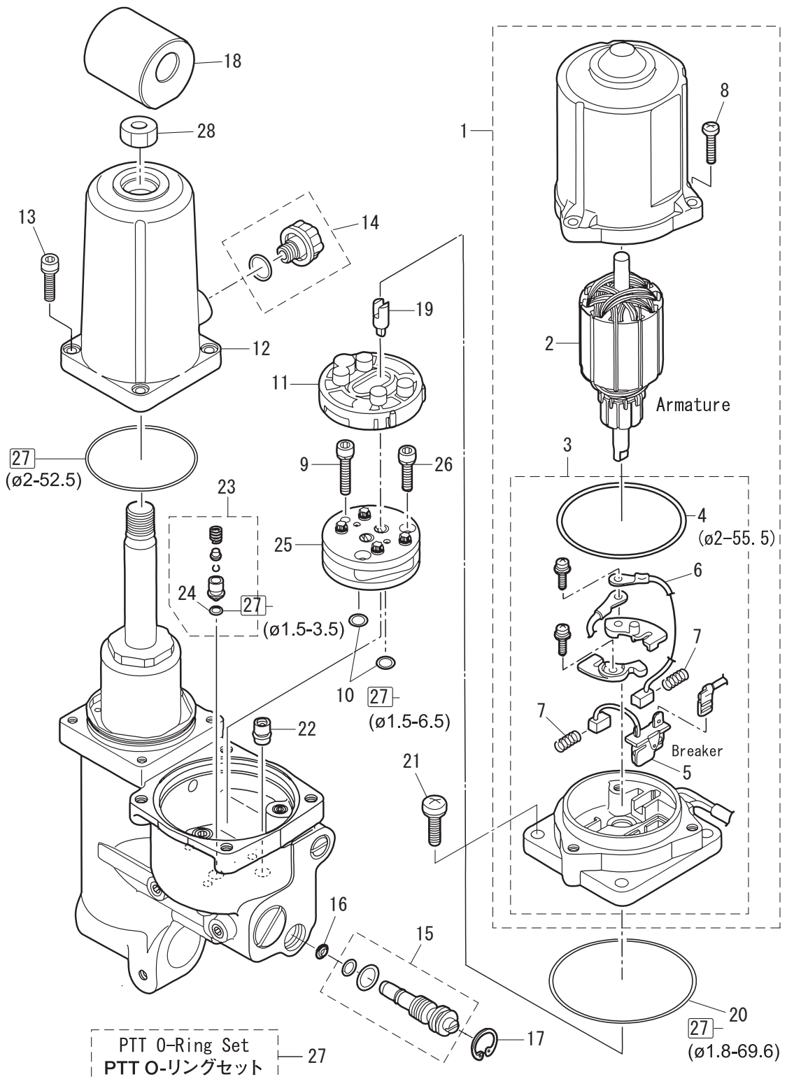
Fig. 14 POWER TRIM & TILT パワートリム & チルト
