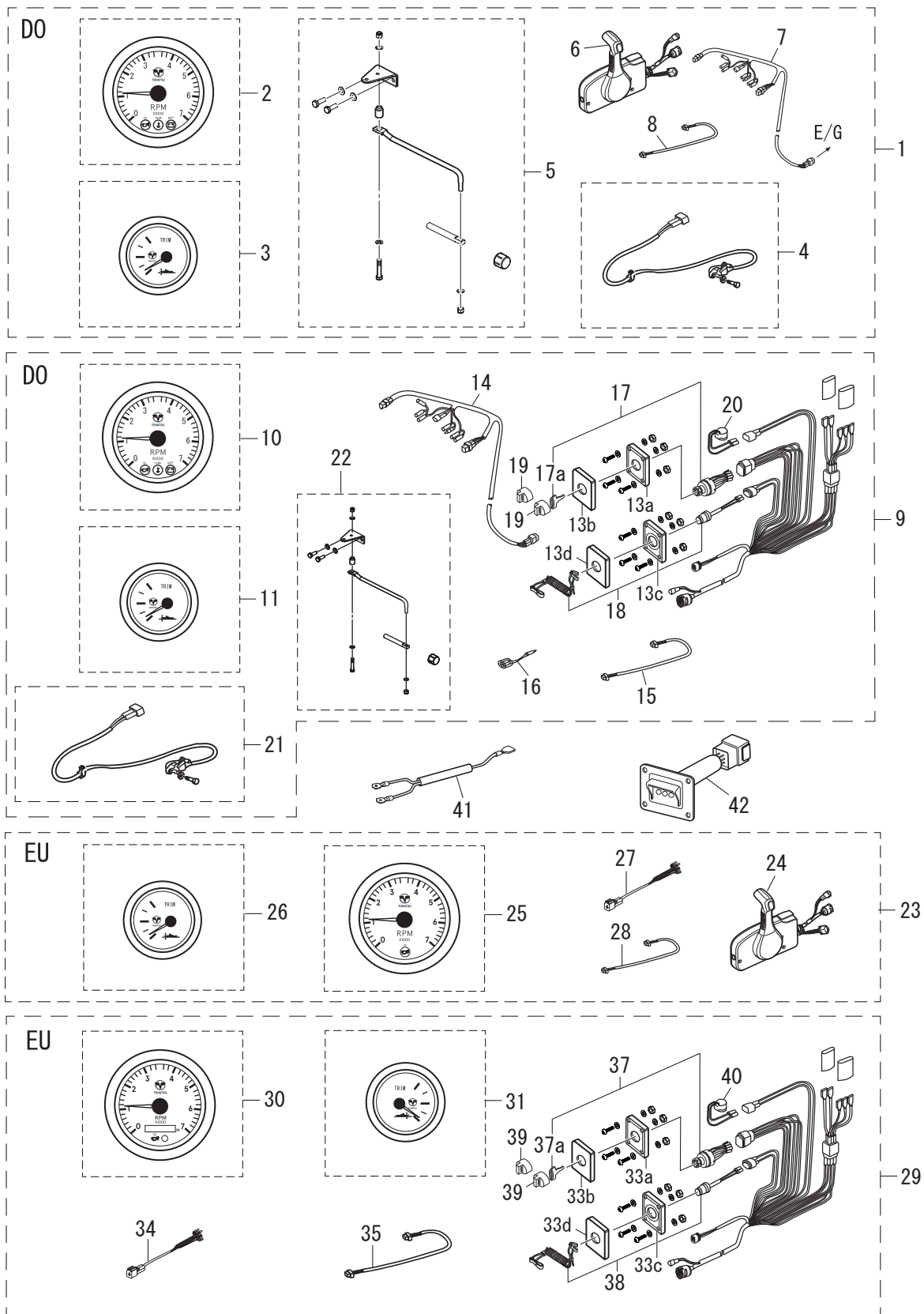
Fig. 25 RIGGING KIT(1) リギングキット (1)
