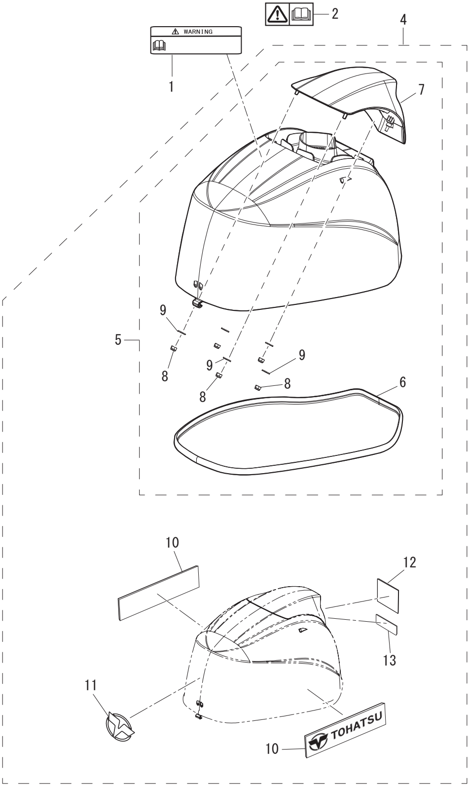
Fig. 18 TOP COWL トップカウル
