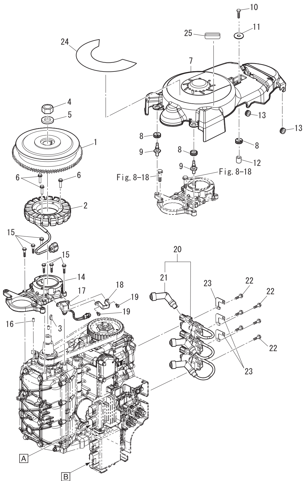
Fig. 7 MAGNETO マグネト
