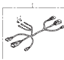
FOP-11 インターフェイスケーブルキット
