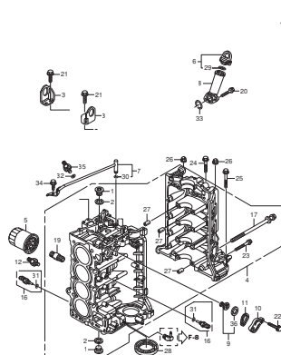
E-3 シリンダーブロック
