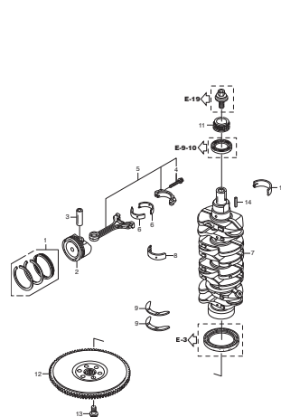
E-7 クランクシャフト/ピストン
