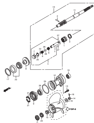
F-5 プロペラシャフト
