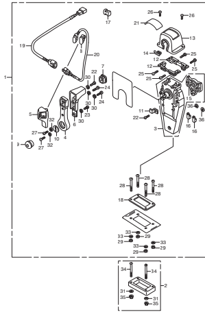
FOP-4 リモートコントロール (トップマウントシングルタイプ) (右)
