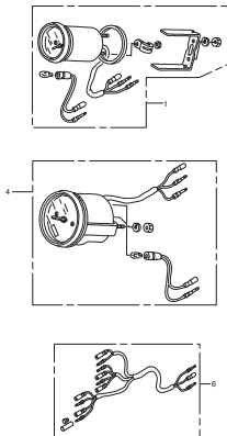
FOP-7 メーター
