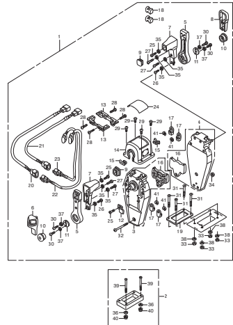
FOP-6-1 スイッチパネルキット (2)
