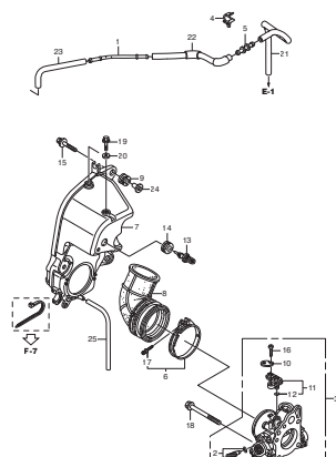
E-18-20 ペーパーセパレーター
