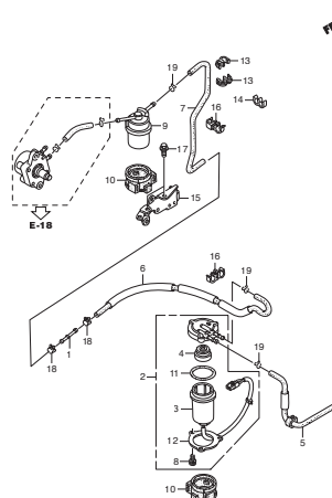
E-18-10 ウォーターセパレーター
