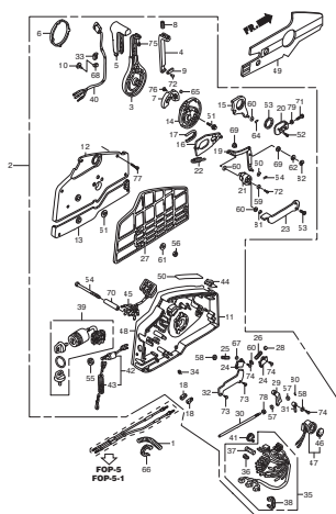
F-15 リモートコントロール (1)
