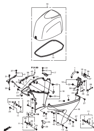
F-8 エンジンカバー/アンダーカバー
