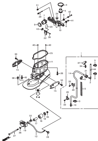
F-3-30 マウントケース
