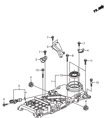
E-9-10 チェンケース
