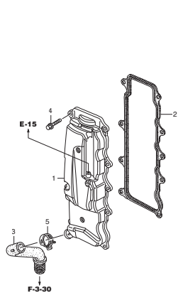
E-1 シリンダーヘッドカバー
