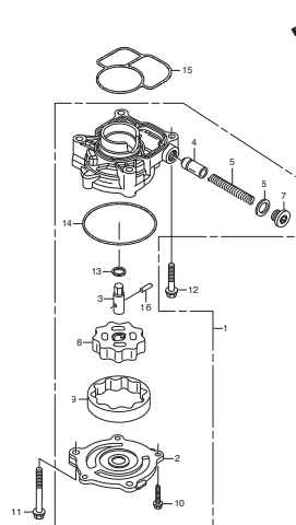
E-5 オイルポンプ
